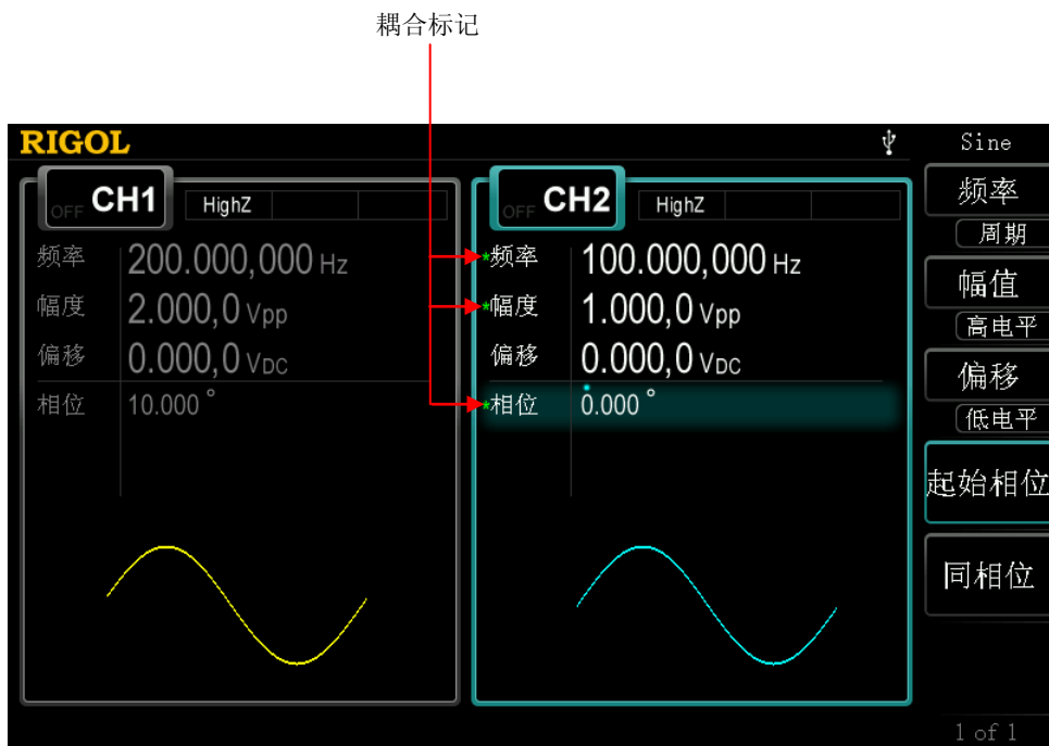
图 10-4 通道耦合
