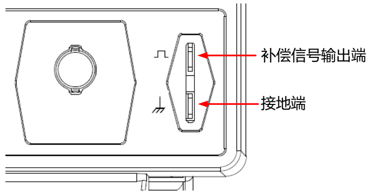
图 4.7 补偿信号
