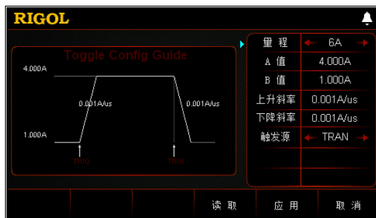
图 2-23 Tog 模式向导界面
