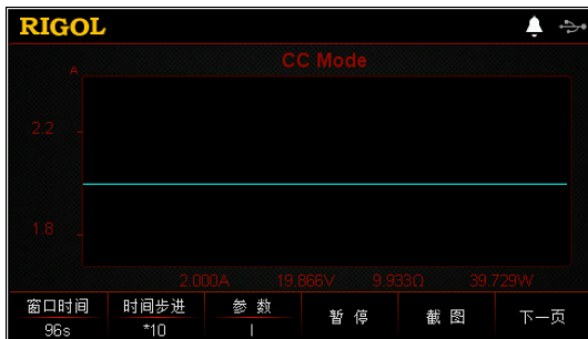
图 2-4 CC 模式波形显示界面
