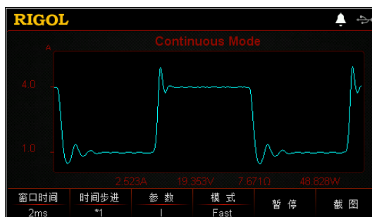
图 2-17 Con 模式波形显示界面
