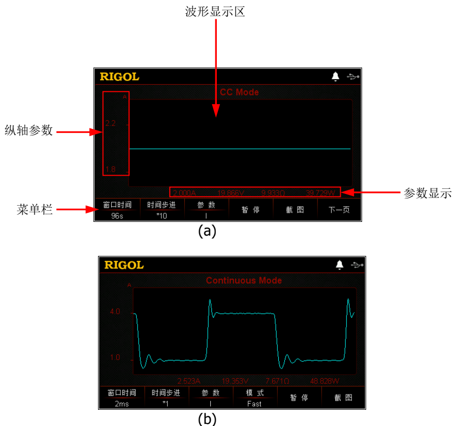
图 2-43 波形显示界面
