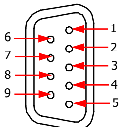
图 2-55 RS232 接口
