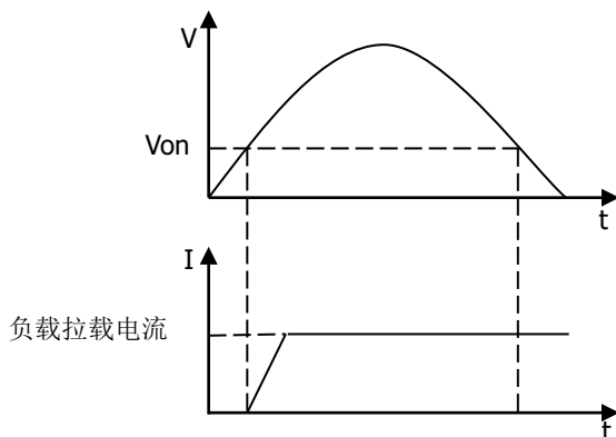
图 2-44 打开 Von Latch 功能
