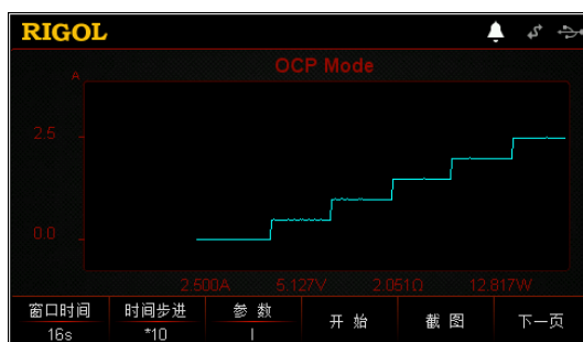
图 2-31 OCP 波形显示界面
