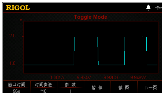
图 2-25 Tog 模式波形显示界面
